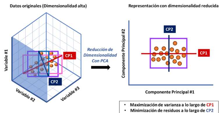
Figura 1.17. Reducción de dimensionalidad con algoritmo PCA.
