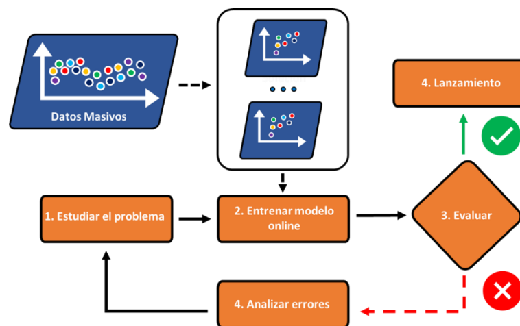
Figura 1.23. Manejo de errores utilizando Aprendizaje en línea.
