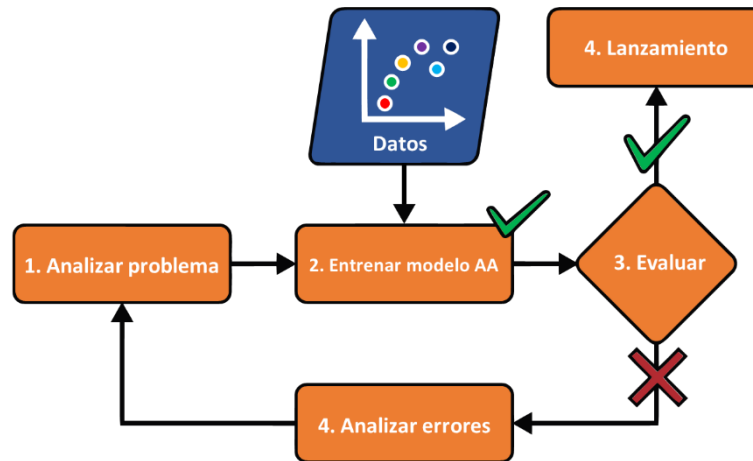
Figura 1.2 Enfoque de Aprendizaje automático
