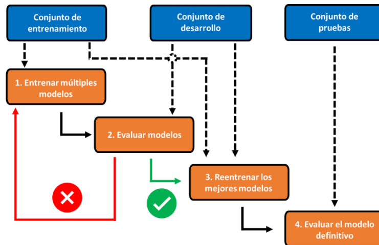
Figura 1.27. Selección de modelos utilizando validación de retención.
