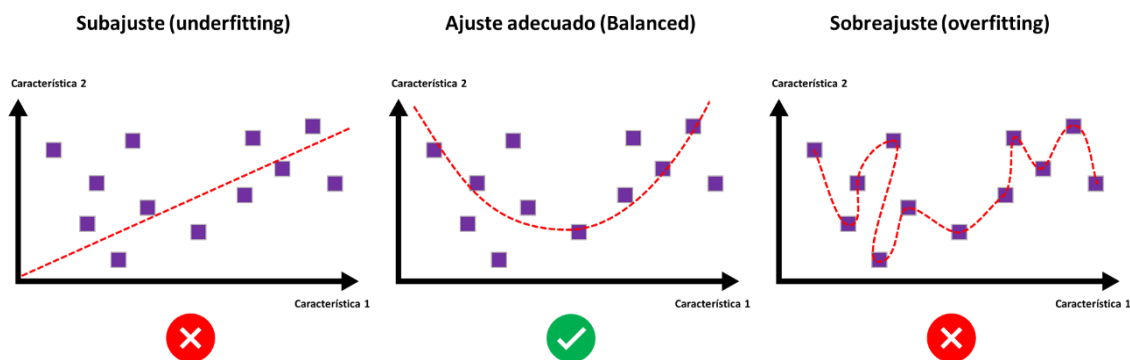
Figura 1.26. Comparativa ajustes de modelos.
