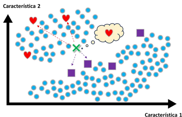
Figura 1.19. Aprendizaje semi-supervisado.
