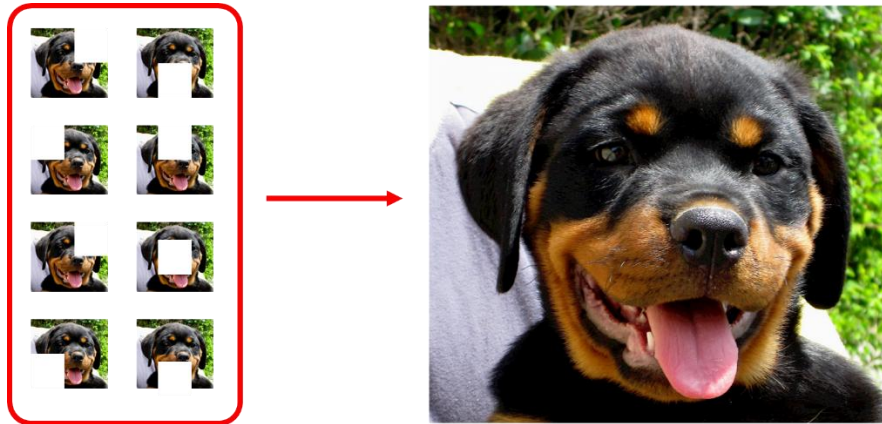
Figura 2.20. Aprendizaje auto-supervisado
