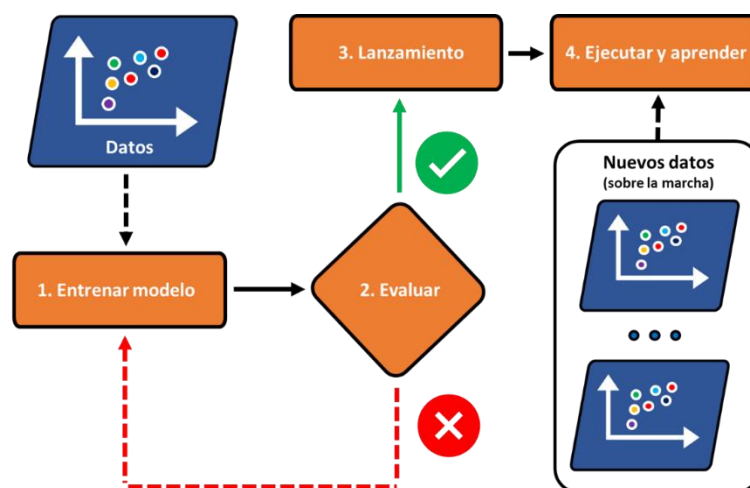
Figura 1.22. Aprendizaje en línea.
