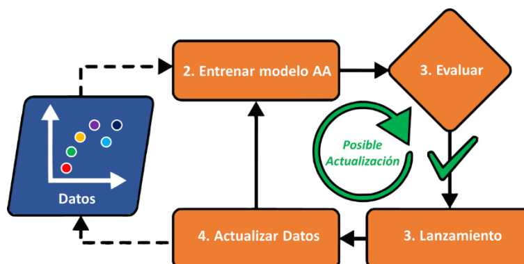
Figura 2.3 Actualización automática a los cambios.
