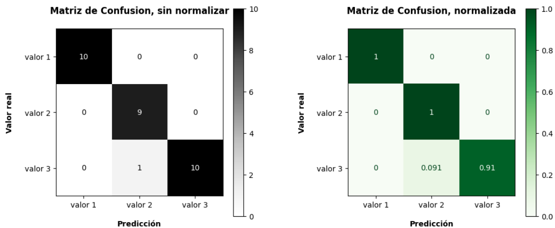
Figura 1.31. Matrices de confusión sin normalizar (izquierda) y normalizada (derecha).
