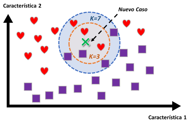
Figura (1.10). Ejemplo de algoritmo K-NN. El valor de "K" indica la cantidad de datos conocidos más cercanos al nuevo caso que se tomarán para realizar la clasificación.
