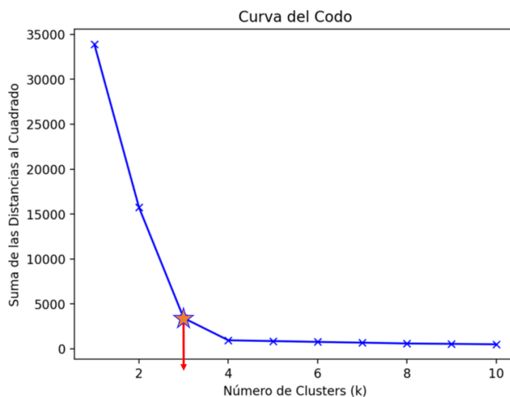
Figura (1.32). Método del codo para obtener el número de clusters óptimo.
