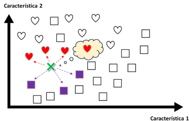
Figura 1.24. Aprendizaje basado en instancias.
