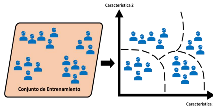
Figura 1.15. Un conjunto de entrenamiento sin etiquetar y un algoritmo de agrupamiento para aprendizaje automático no supervisado
