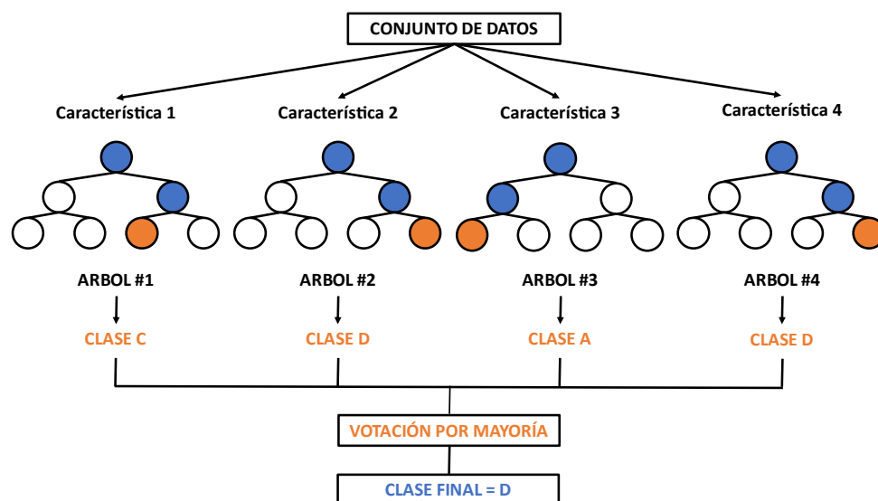
Figura (1.11). Random Forest utiliza el método de bagging para el entrenamiento (y combinación) de modelos y la votación por mayoría para llegar al consenso.
