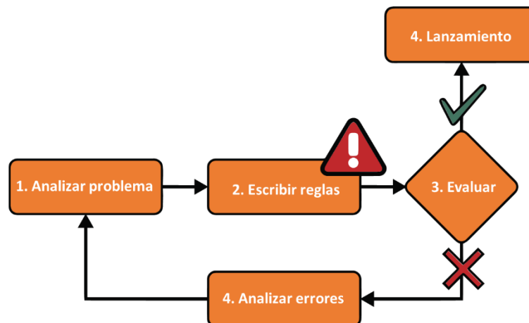
Figura 1.1 Enfoque tradicional
