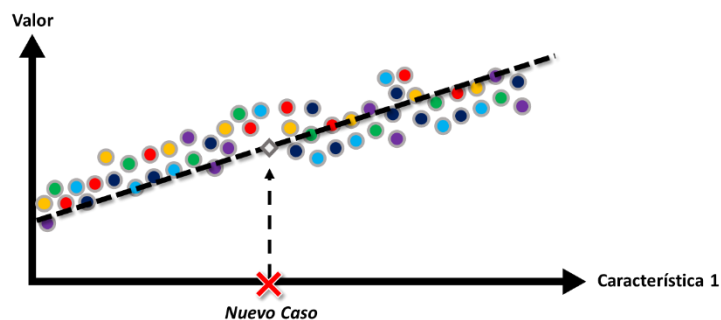
Figura 1.13. Regresión lineal.
