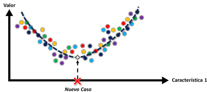
Figura 1.14. Regresión Polinómica.
