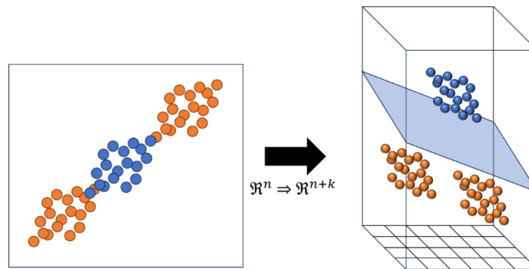
Figura (1.8). Solución de un problema de clasificación no linealmente separable en dos dimensiones mediante el uso de SVM para aumentar su dimensionalidad.
